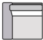
B150L 132 cm x 83 cm x110 cm 42 kg / 1 pcs vol. 1,21 m 3
